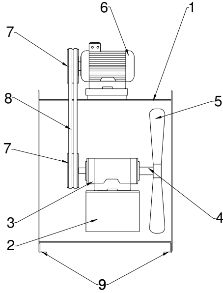
Şekil 3 : Kayış - Kasnak Tahrikli Aksiya Vantilatör
