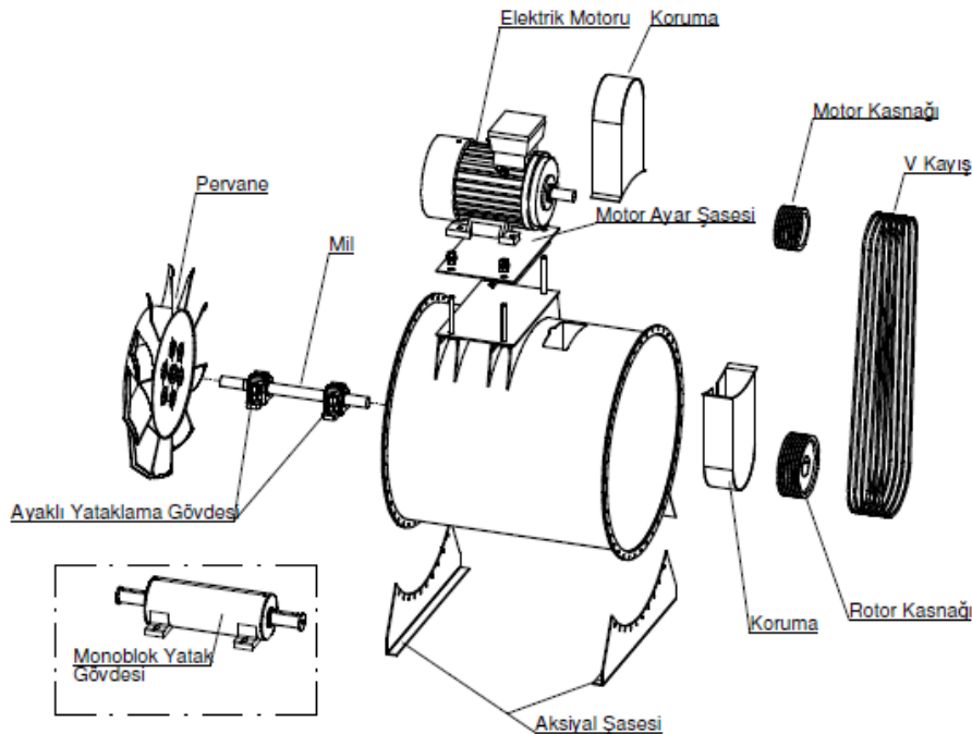
Şekil 8 : Pervane, Yatak ve Rulmanların değiştirilmesi
