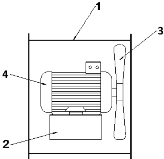
Şekil 2 : Motor Direk Akuple Aksiya Vantilatör
