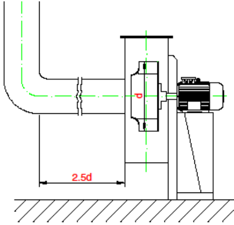
Şekil 6 : Emiş kanalı ile minimum kurulum uzaklıkları
