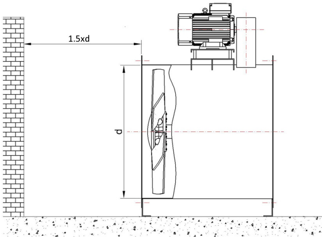
Şekil 7 : Serbest emiş ile minimum kurulum uzaklıkları
